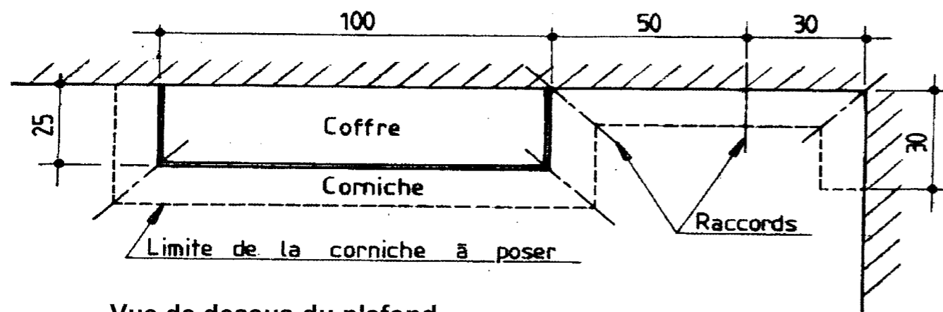
Vue de dessus du plafond
